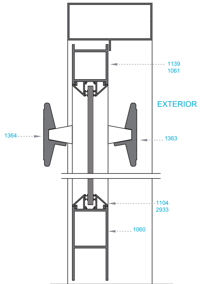
SECCIÓN HORIZONTAL (B - B)
