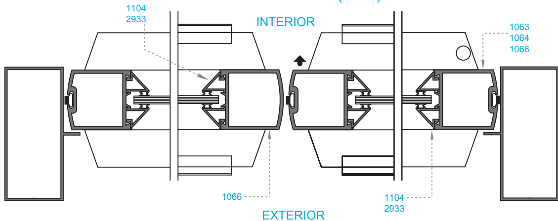
SECCIÓN HORIZONTAL (B - B)
